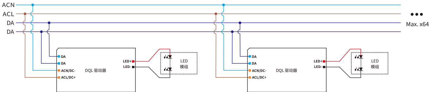
接线图
