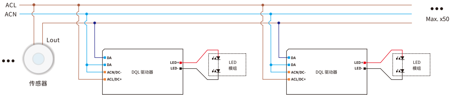
接线图
