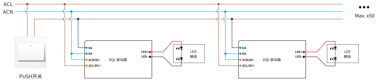
接线图
