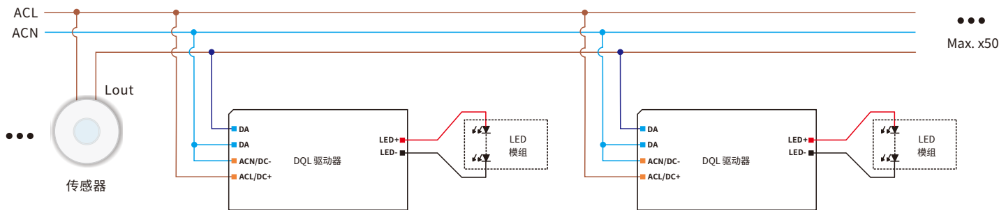
接线图
