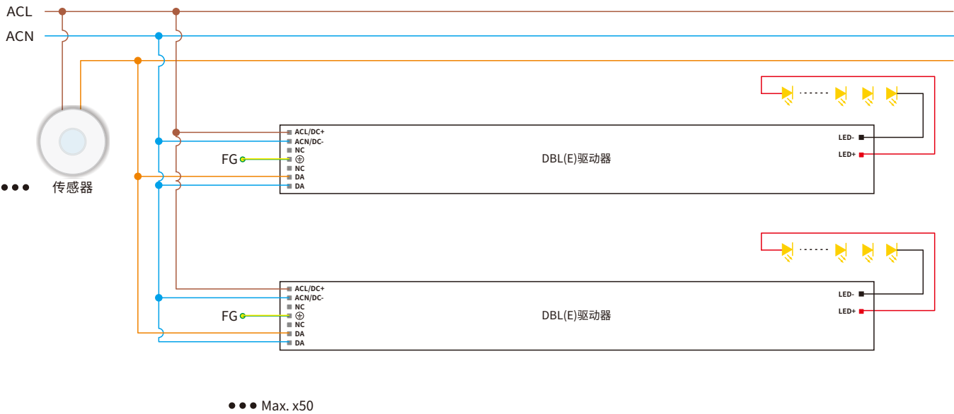
接线图
