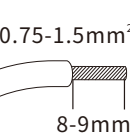
输入线材
