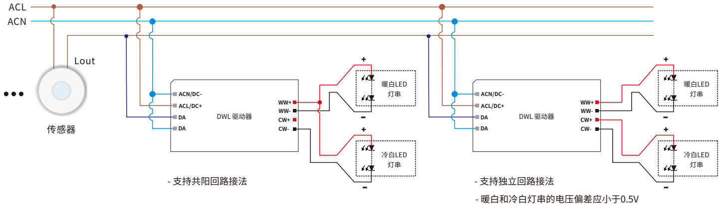
接线图
