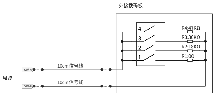
4档接线图
