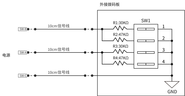
16档接线图
