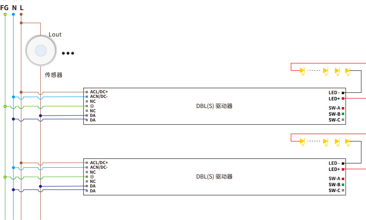
接线图
