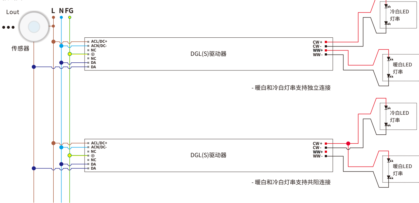
接线图
