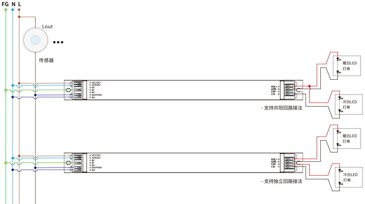
接线图
