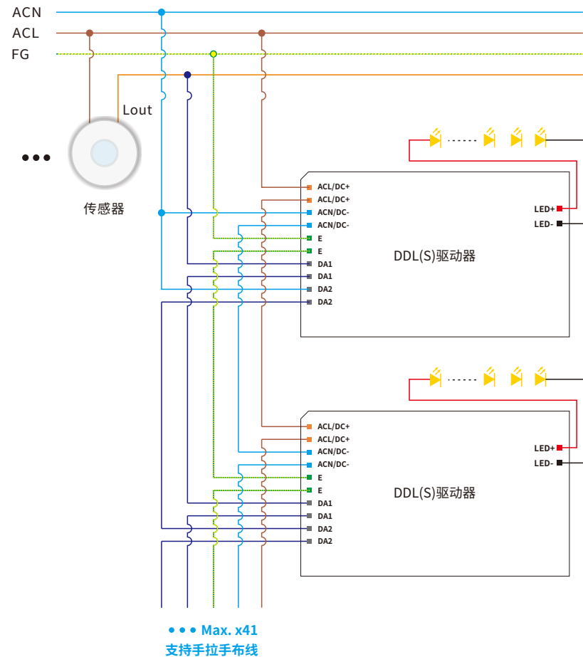
接线图
