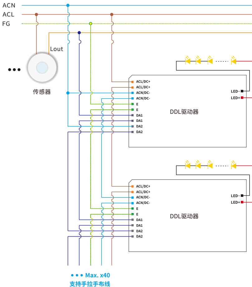
接线图
