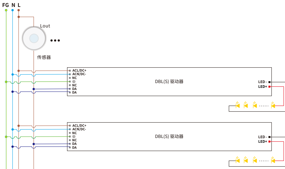
接线图
