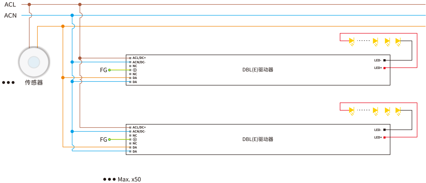
接线图
