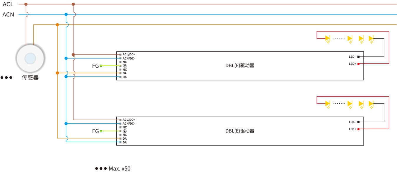
接线图
