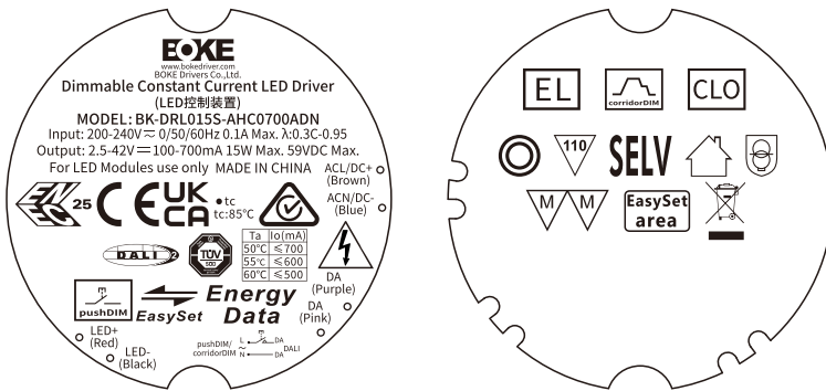
镭雕工艺
