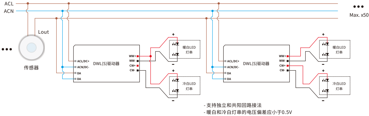
接线图
