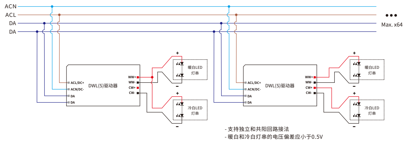
接线图
