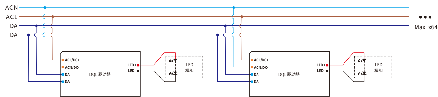
接线图
