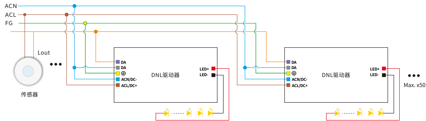
接线图
