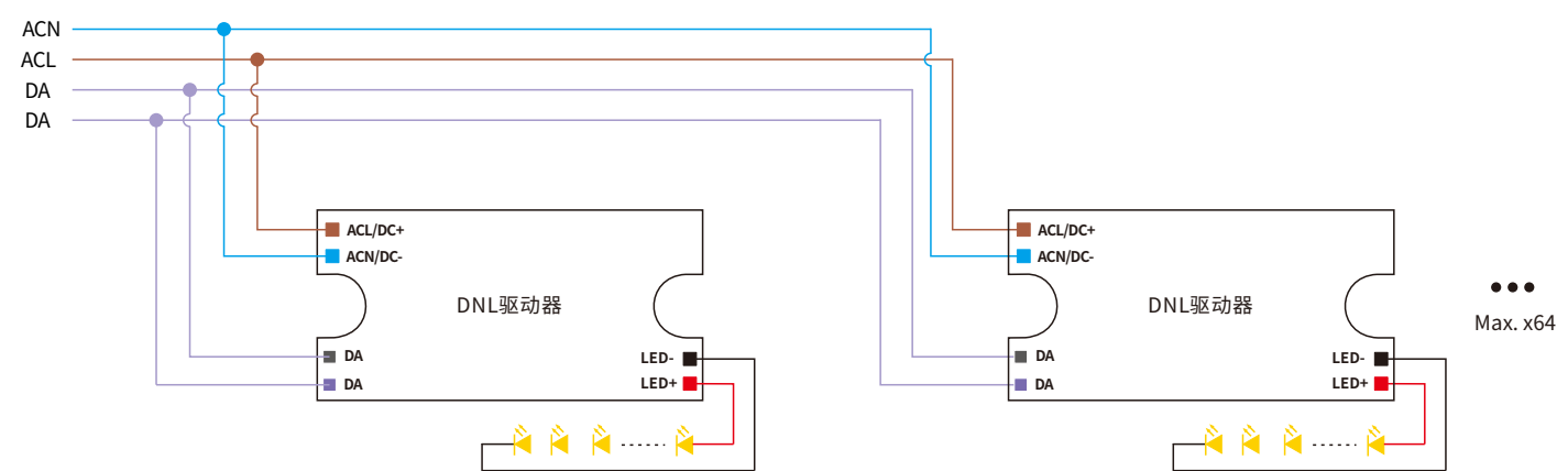
接线图
