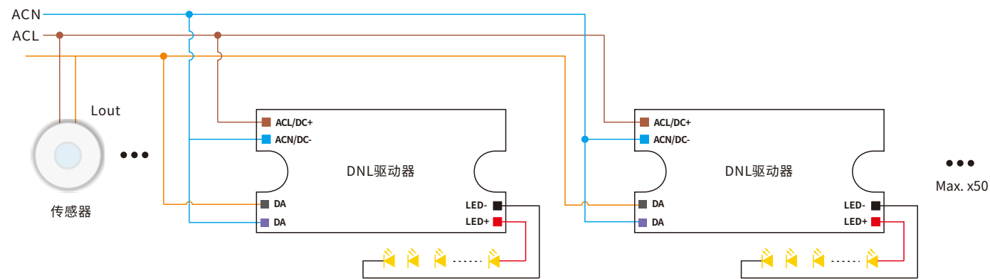
接线图
