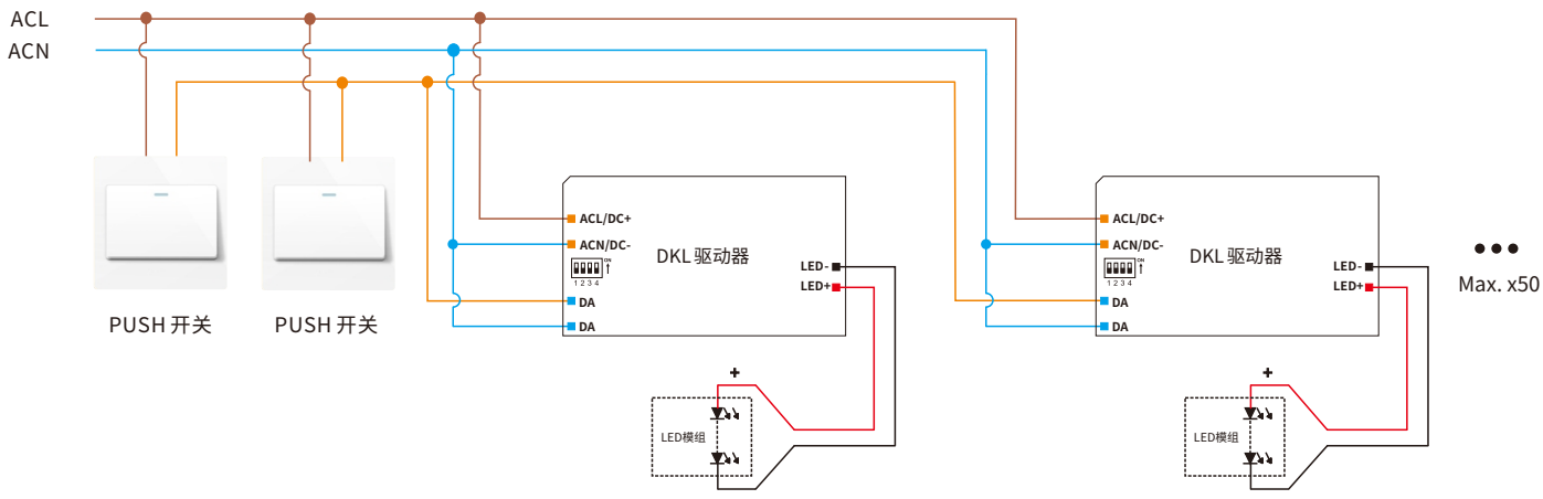
接线图
