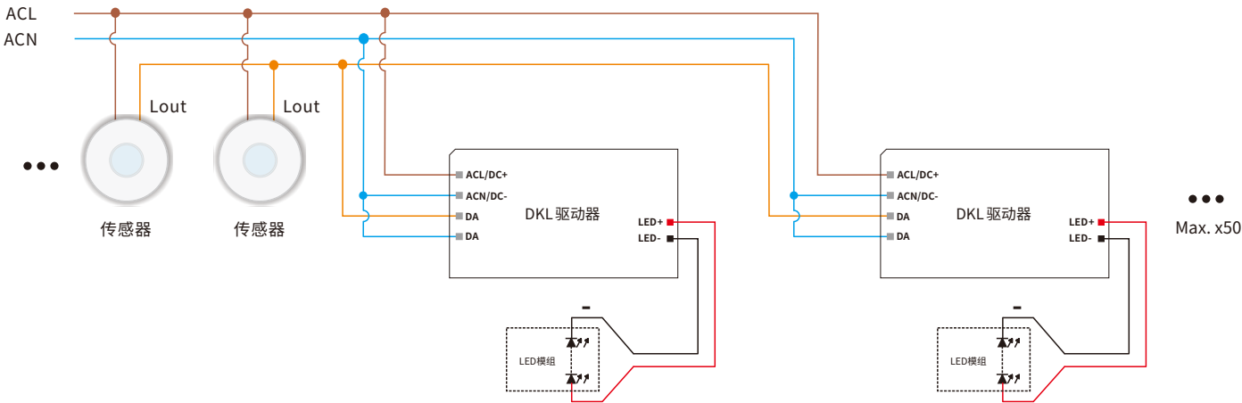
接线图
