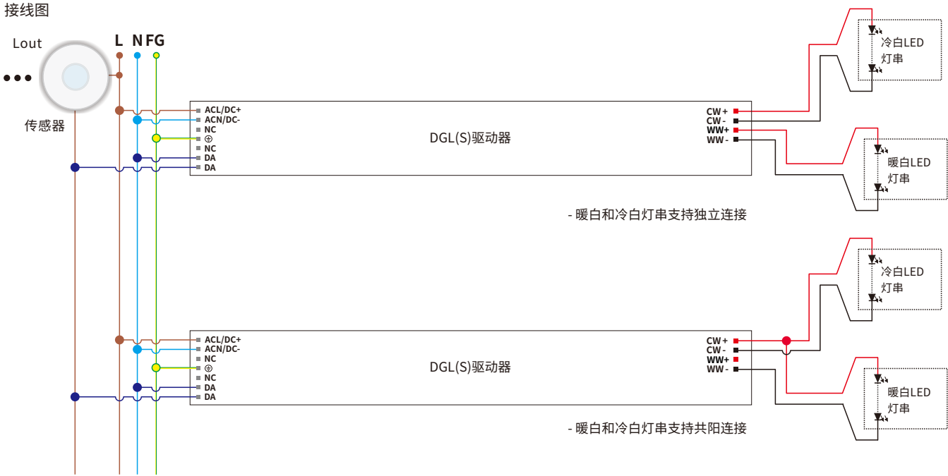
接线图
