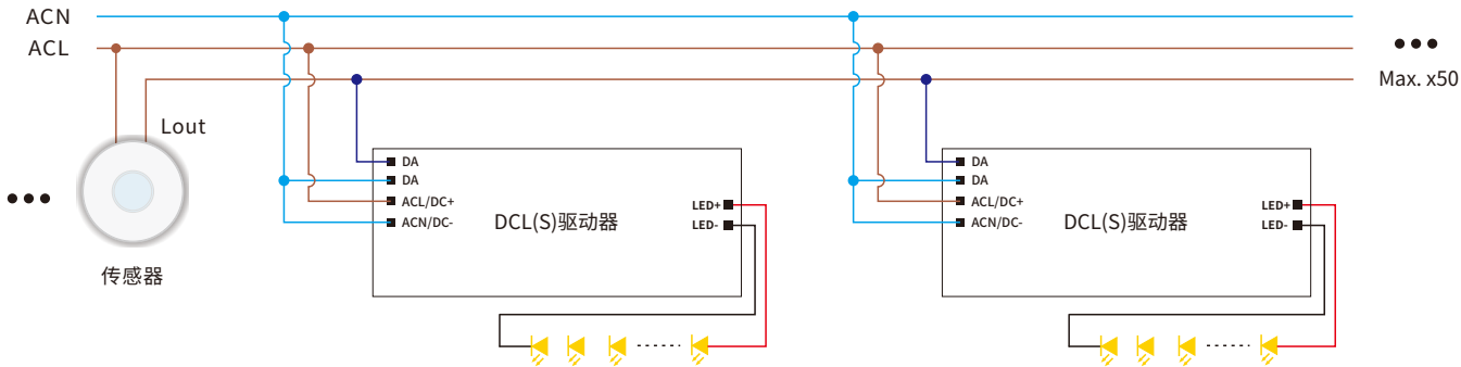
接线图
