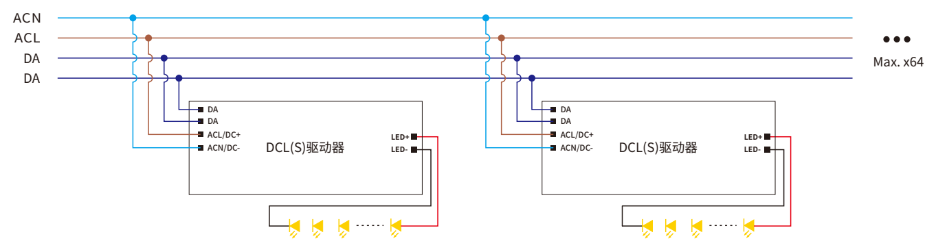
接线图
