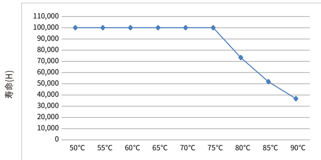
寿命 vs. 外壳温度
