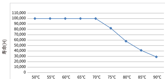
寿命 vs. 外壳温度
