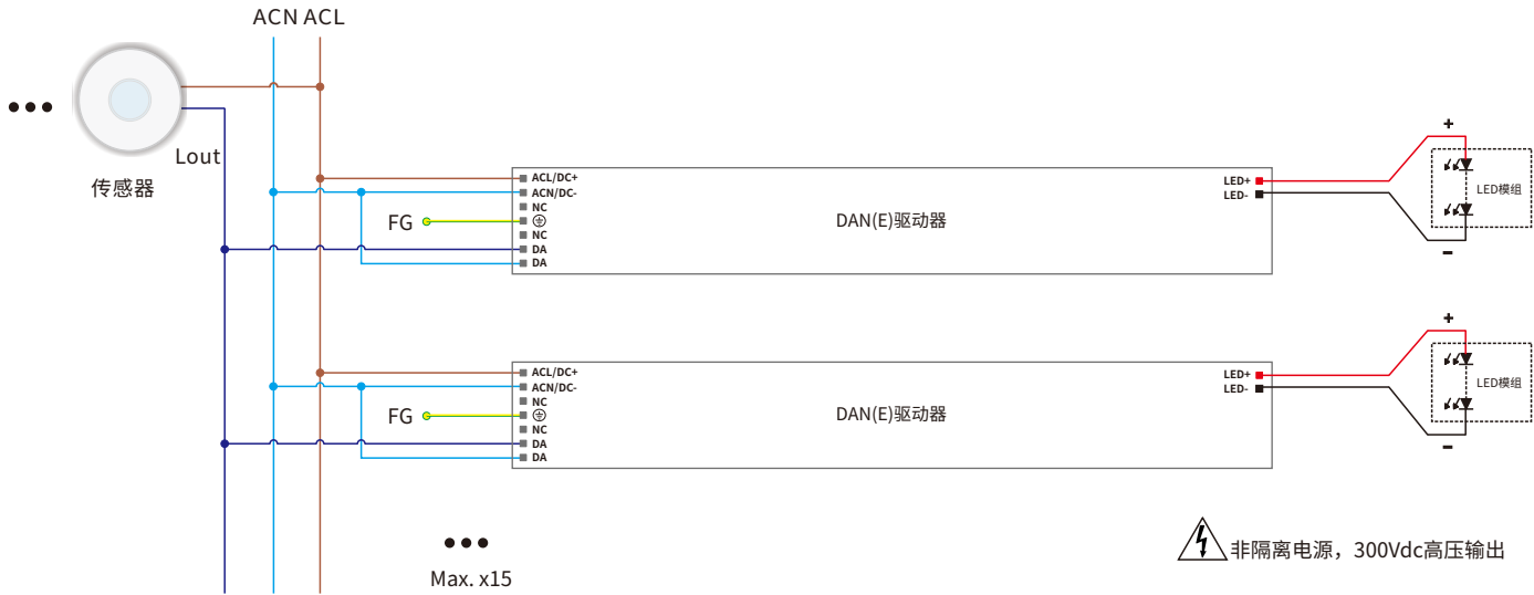
接线图
