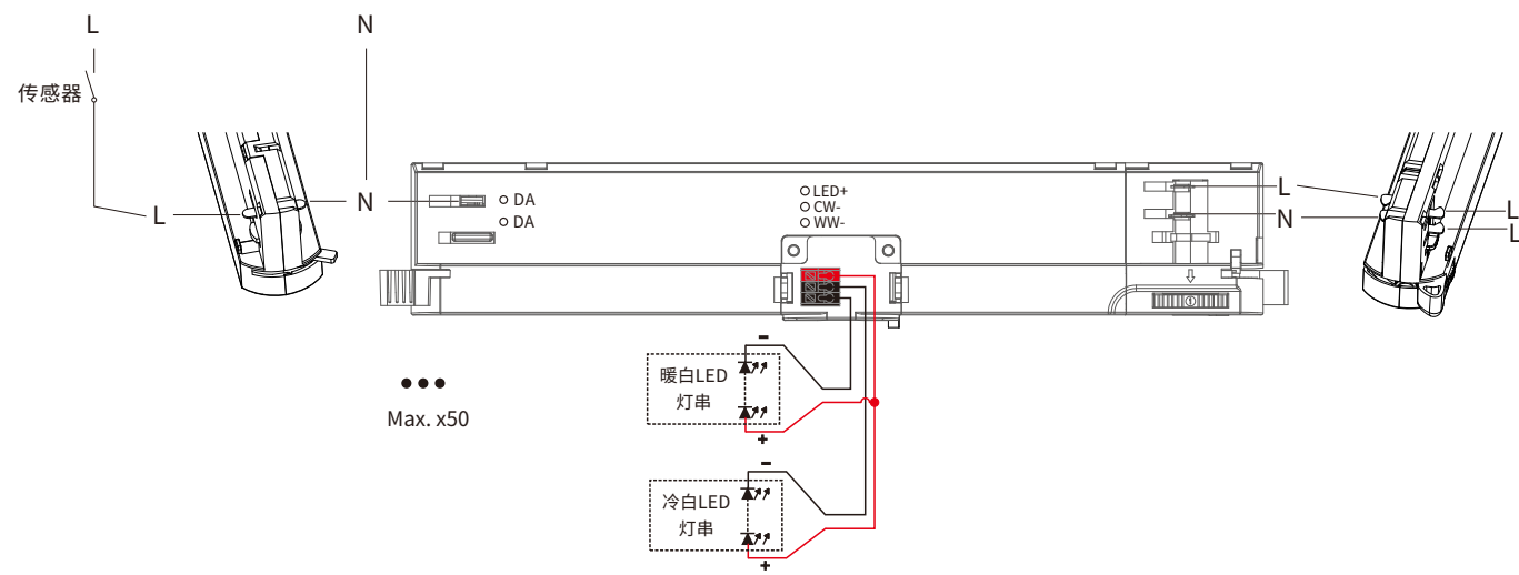
接线图
