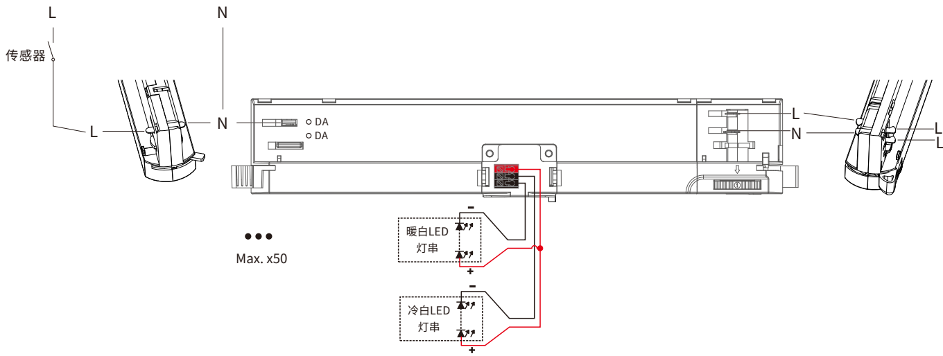
接线图
