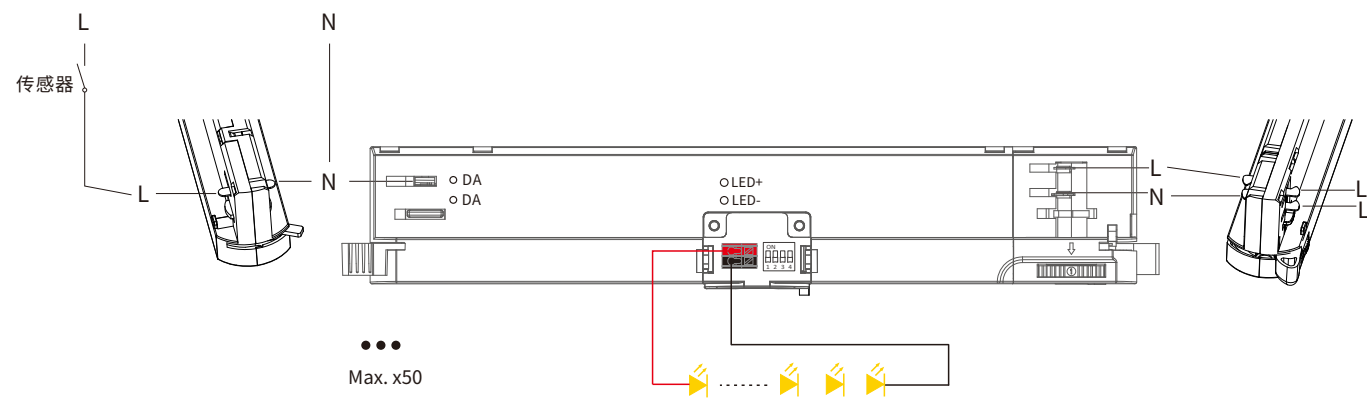
接线图
