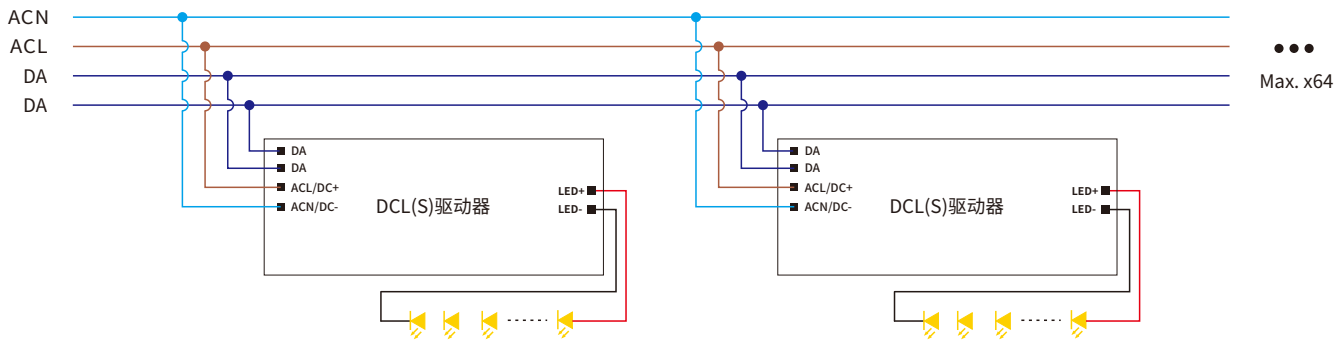
接线图
