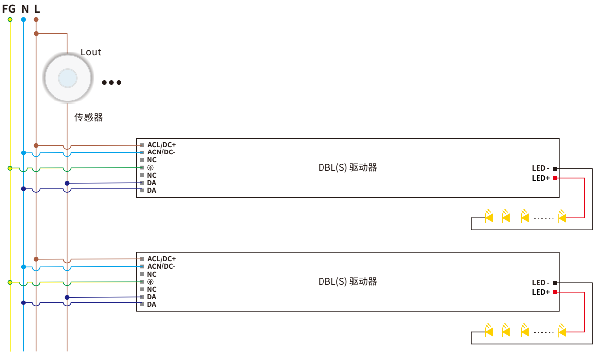
接线图
