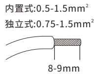
输入线材
