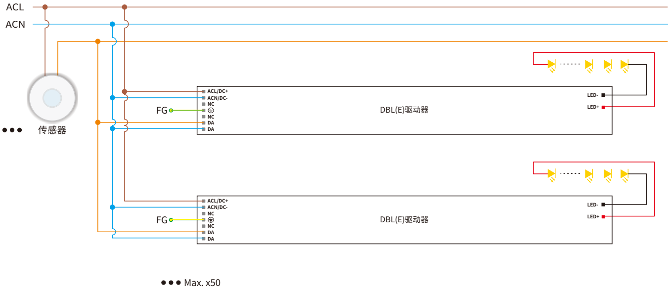
接线图
