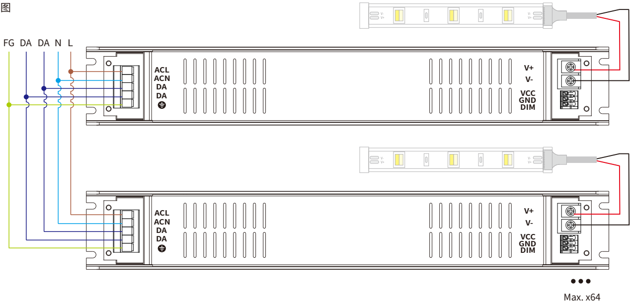
接线图
