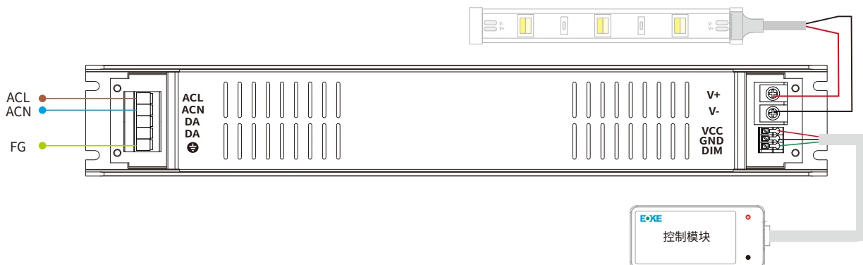
接线图
