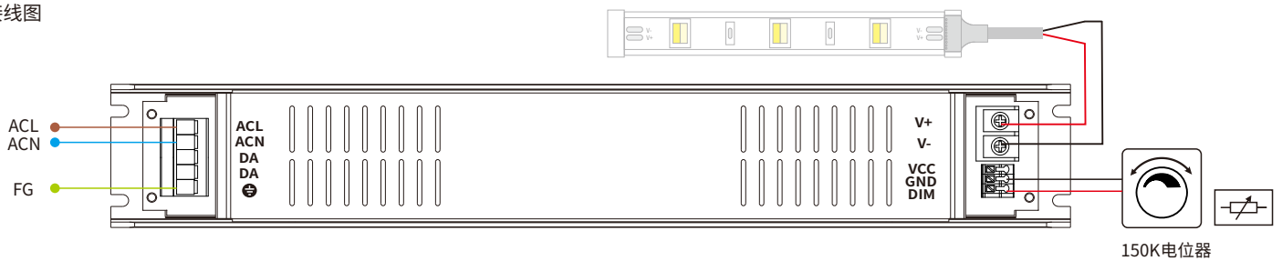
接线图
