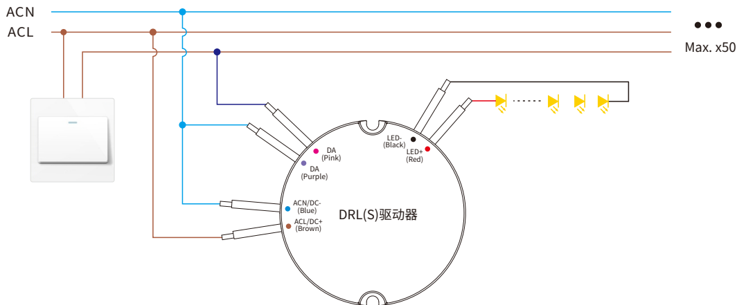
接线图
