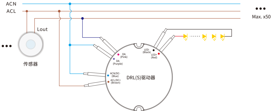
接线图
