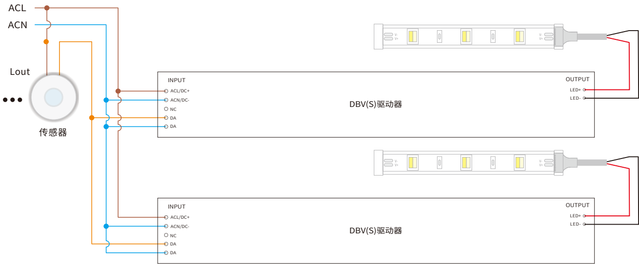
接线图
