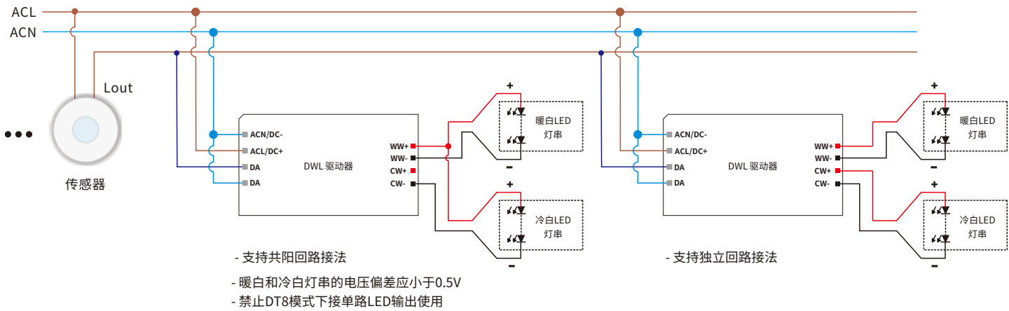
接线图
