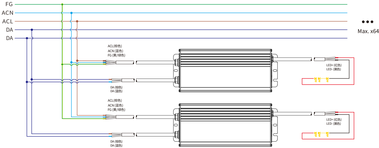
接线图
