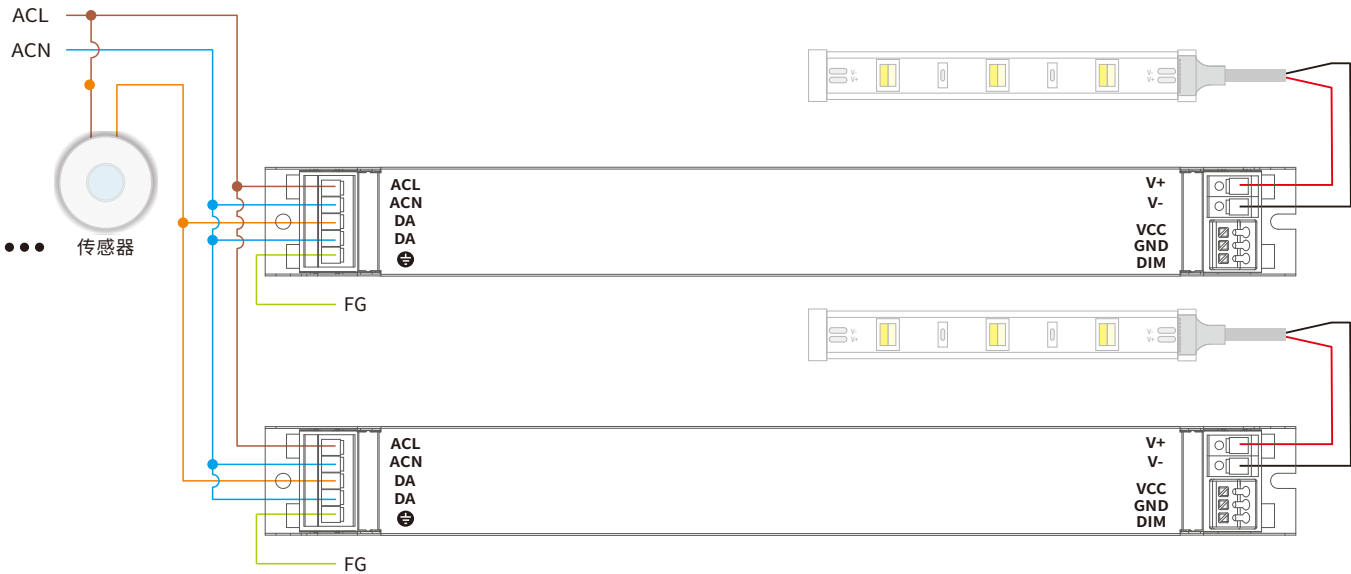
接线图
