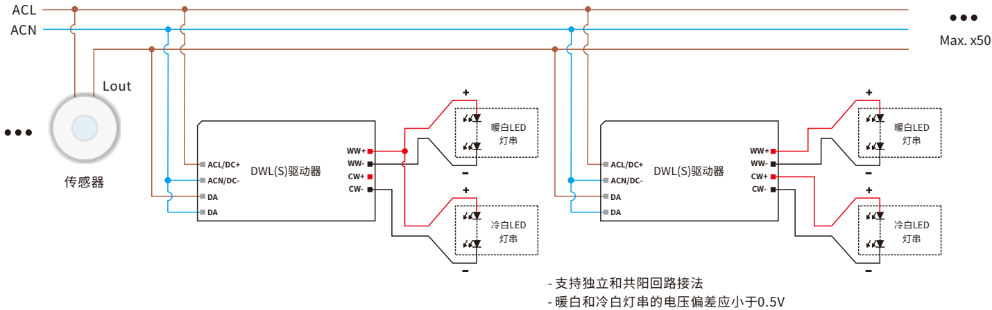
接线图
