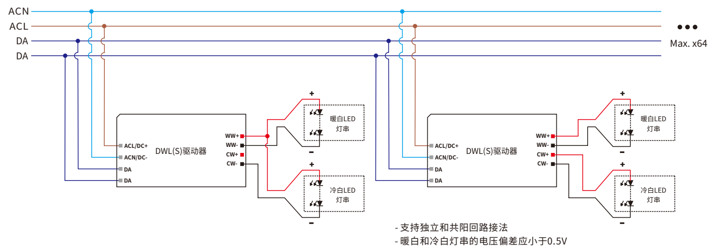
接线图
