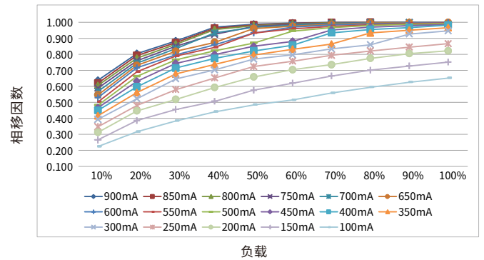
相移因数 vs. 负载
