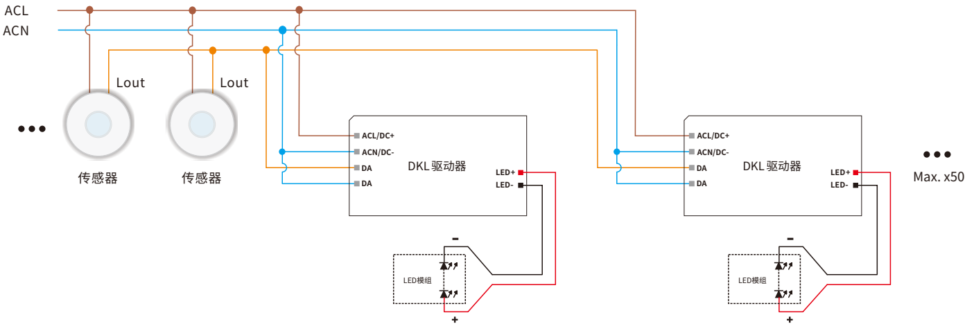
接线图
