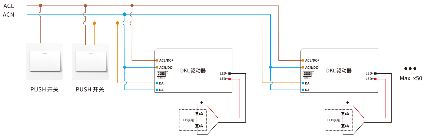
接线图
