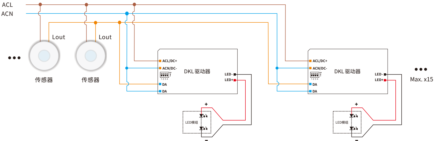
接线图
