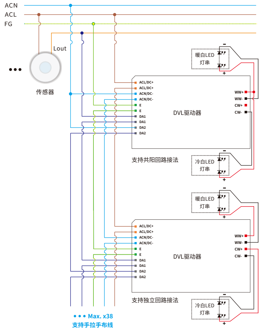
接线图
