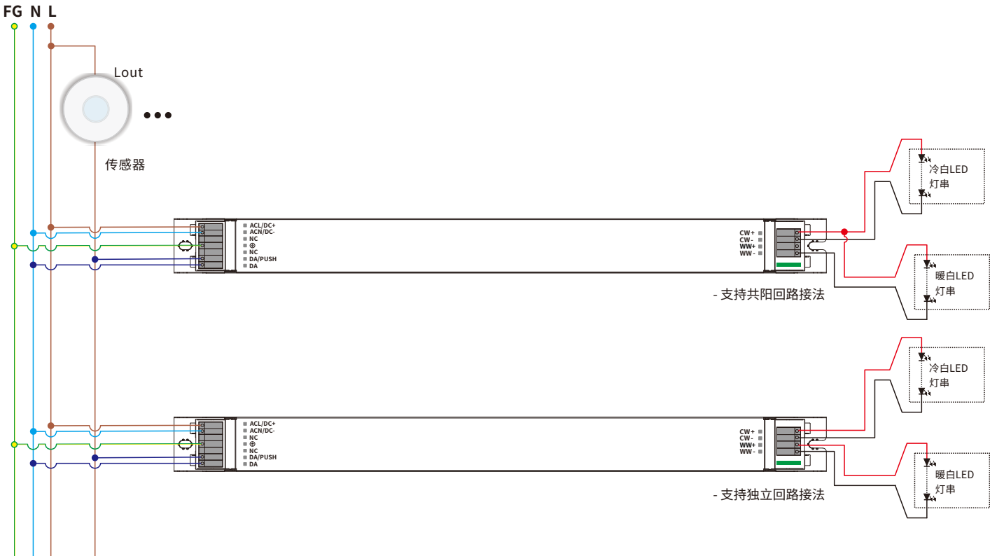
接线图
