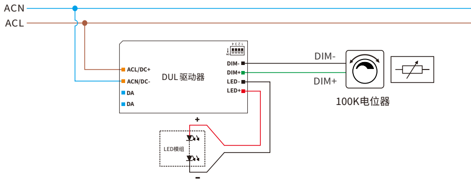
接线图
