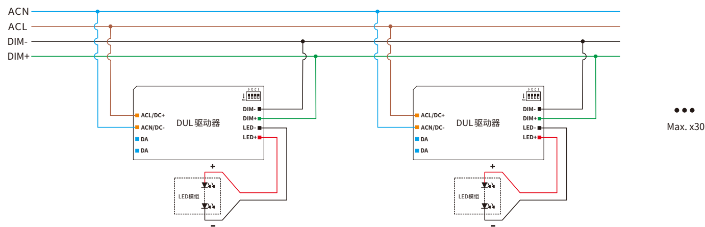
接线图
