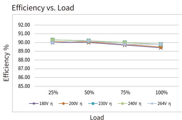
BK-LGV036A-24V0 电气特性曲线图
