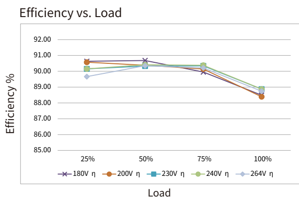
BK-LGV060A-24V0 电气特性曲线图
