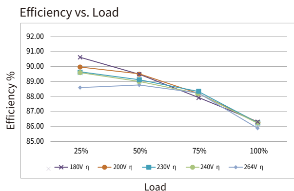
BK-LGV060A-12V0 电气特性曲线图
