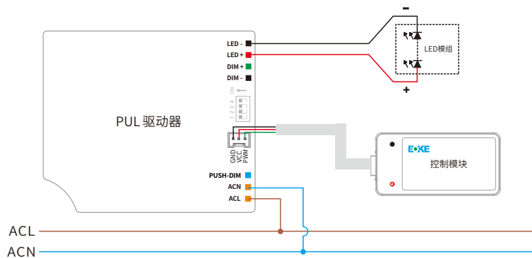
接线图
