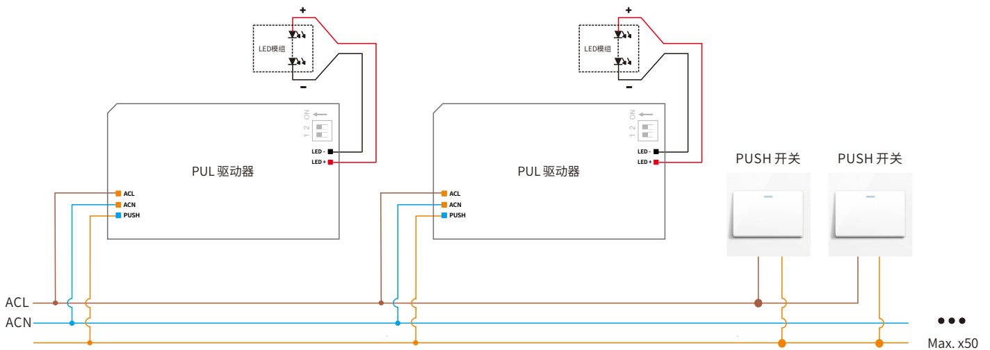
接线图
